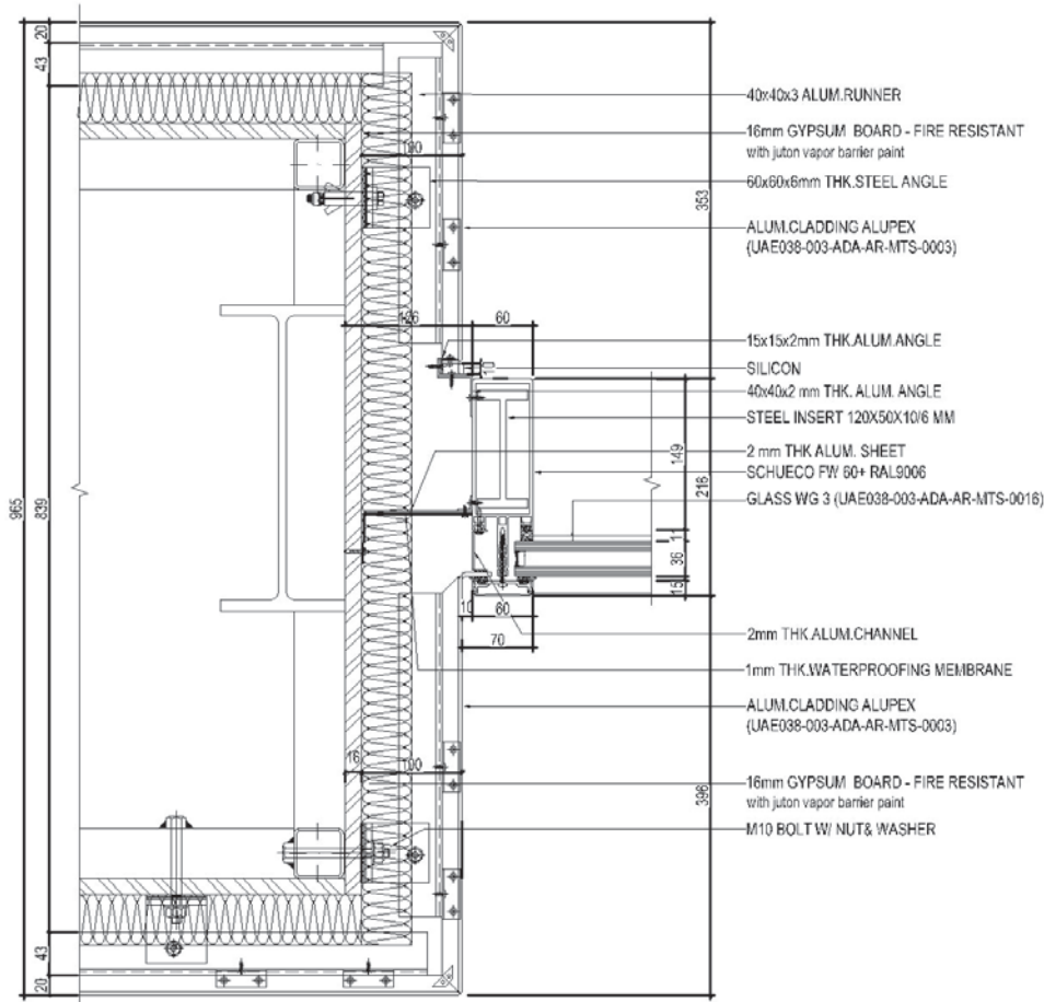
MULLION JAMB DETAIL
