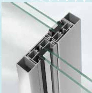
ASE 70 PD ME
